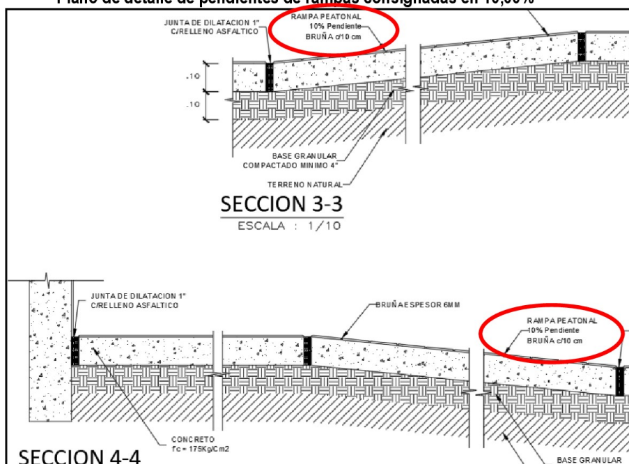
Imagen N° 2 Plano de detalle de pendientes de rampas consignadas en 10,00%
