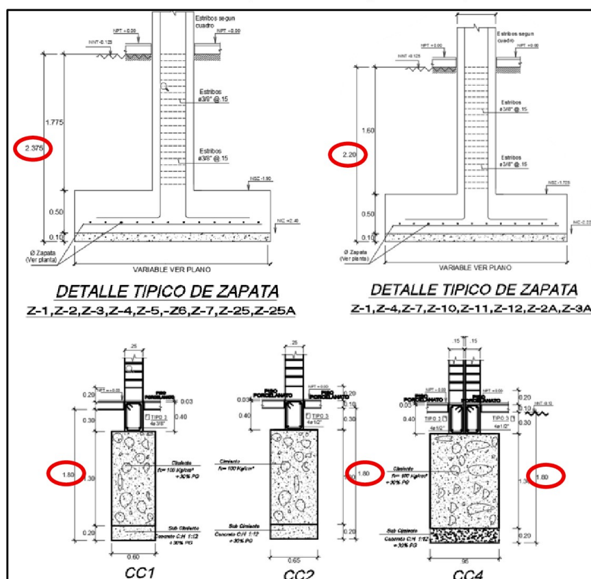
Imagen N° 1 Profundidad de cimentación planteada en los planos del expediente técnico
