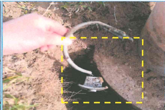
Descripción: Portafusible cortocircuitado
