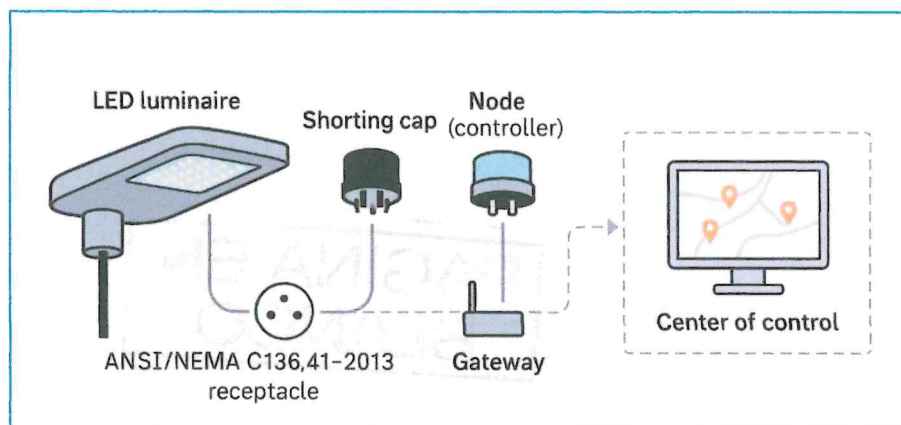
IMAGEN N° 3 SISTEMA DE TELEGESTIÓN EN LUMINARIAS LED
